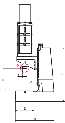
DA Type
